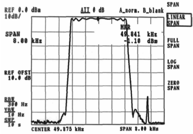
CURVA BANDA PASSANTE
