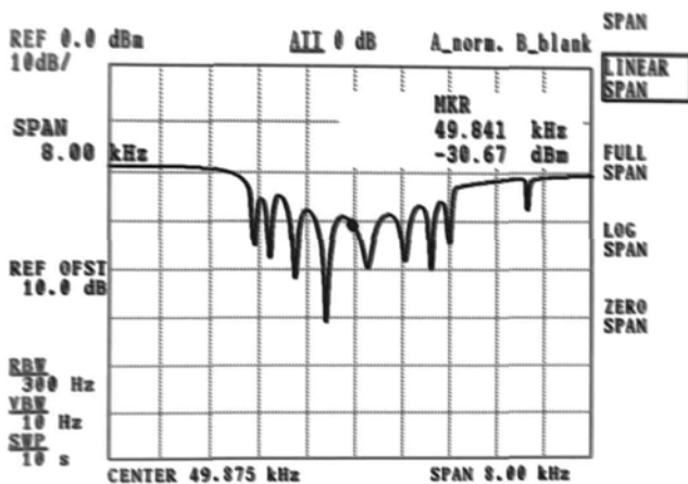
CURVA "RETURN LOSS"
