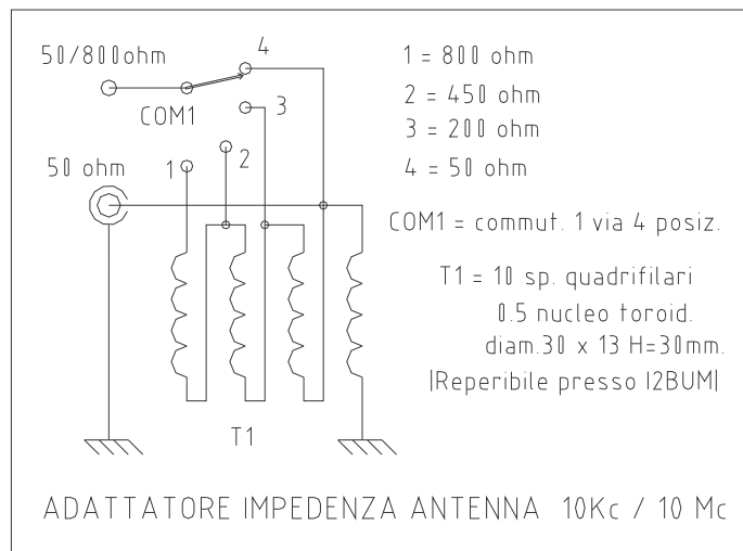
Schema elettrico
